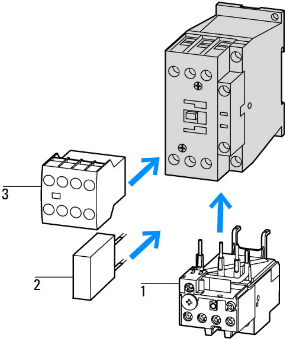
1: Ochronny przekaźnik silnikowy 2: Układ ochronny 3: Moduły wyłącznika pomocniczego
