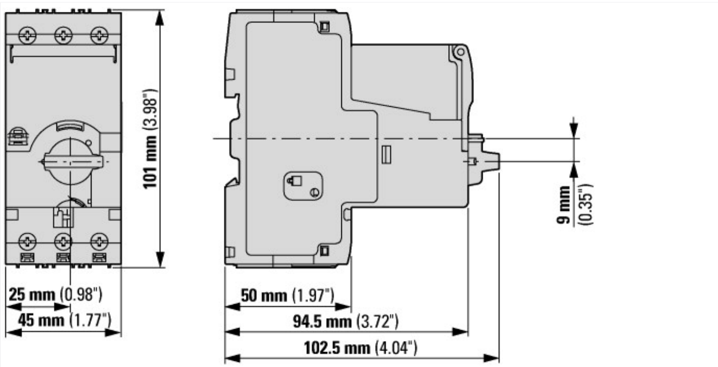
Aparat podstawowy z blokiem wyzwolenia
